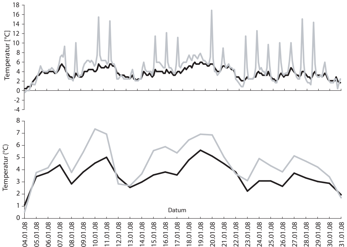
Abb. 5: Temperaturmessungen im Untersuchungsgebiet Chilchberg in der obersten Streuschicht während der Fangperiode G (04.1.2008 - 31.01.2008), jeweils in 5 m Abstand zum Hügelskamm: Schwarze Linie = Nordhang, graue Linie = Südhang; oben: Temperaturkurven (Messung im 3 Stunden Intervall), unten: Tagesdurchschnittswerte.
